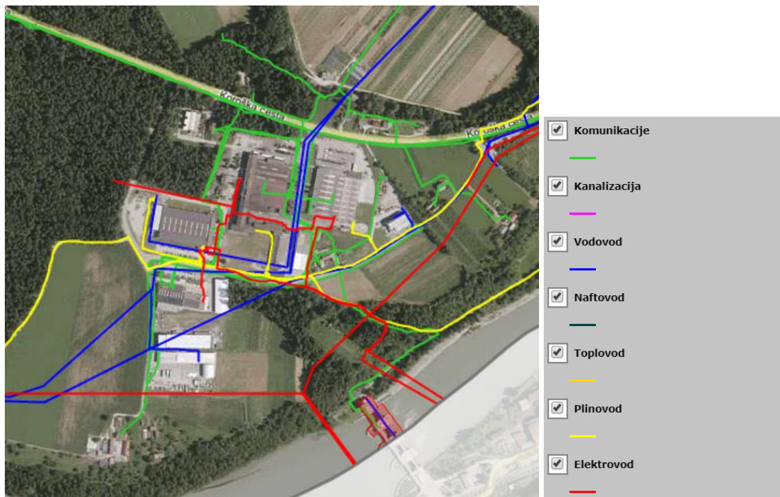
Slika 2: Obstoječa infrastruktura na območju IC Muta.
