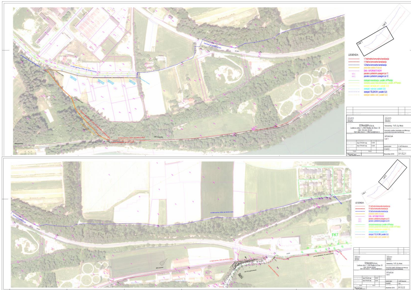
Prikaz izvedbe fekalne kanalizacije – povezovalni vod
