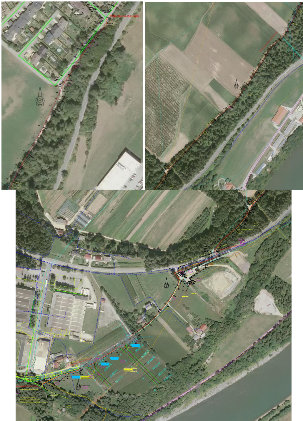
Slika 7: Prikaz tlačnega povezovalnega kanalizacijskega voda
